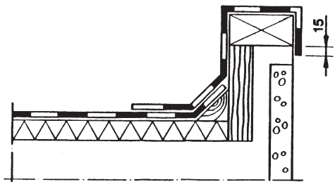
Kuva 4. Räystäs, 1-kermikate.
