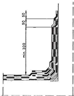
Kuva 9. Seinällenosto, 3-kermikate.
