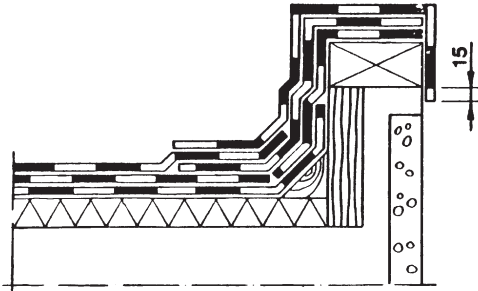
Kuva 6. Rästäs, 3-kermikate.
